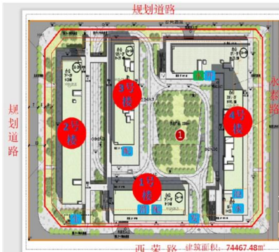
图 2.1 项目平面位置
