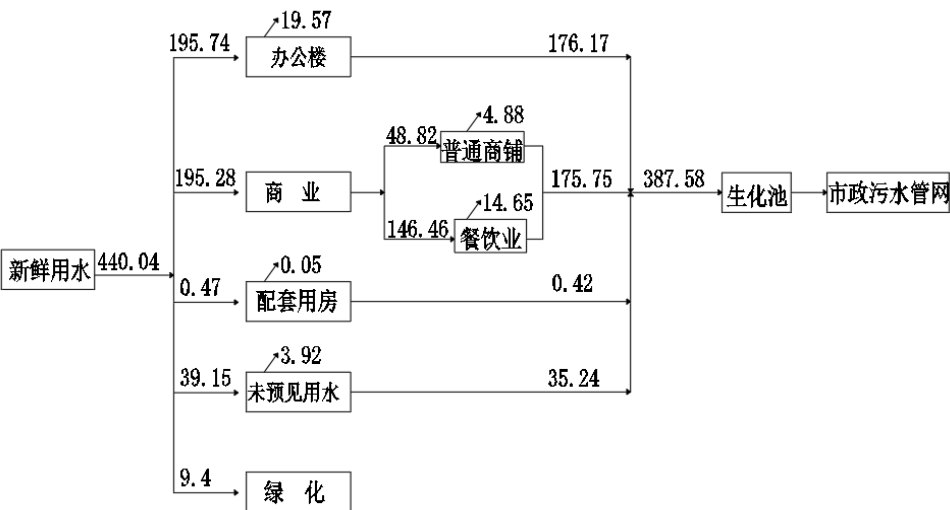
图 2.2 水平衡图（单位：m³/d）
